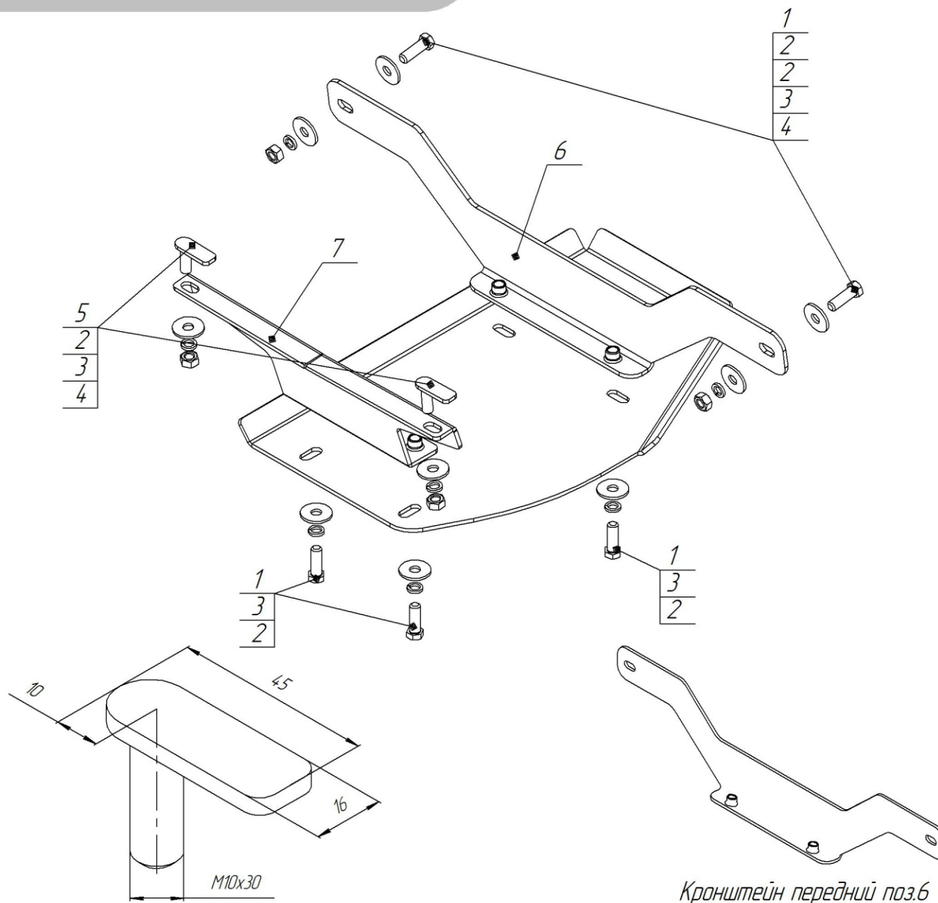
Закладной кронштейн M10x30 поз.5
