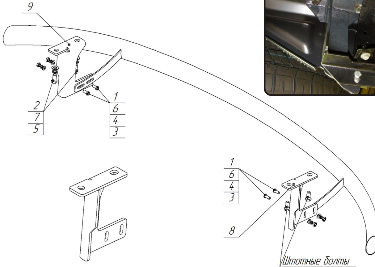
Кронштейн левый (поз.8) правый - зеркальный
