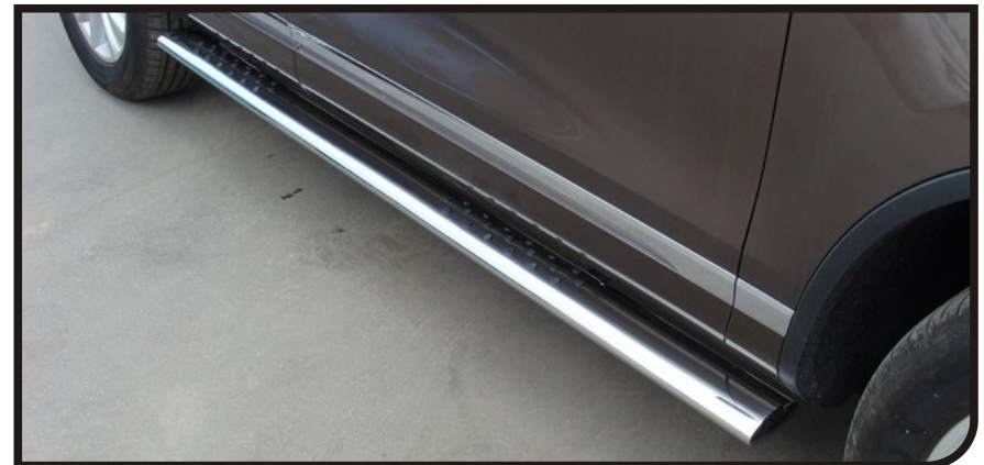
Пороги овальные с проступью 120x60 мм арт. HYUNSF-04 / HYUNSF10-09 / HYUNSF11-09
